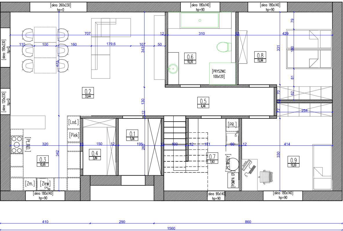
RZUT PARTERU
