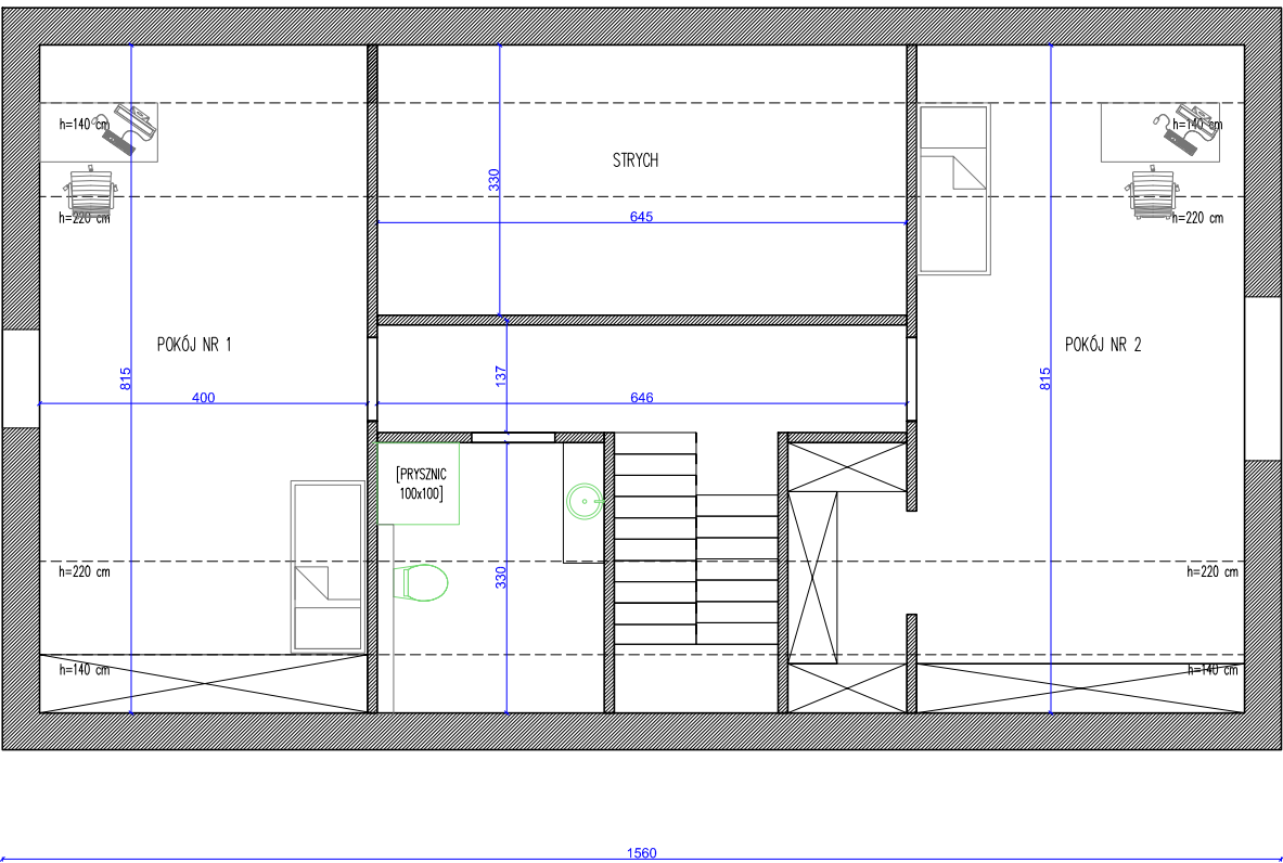
RZUT PODDASZA UŻYTKOWEGO
