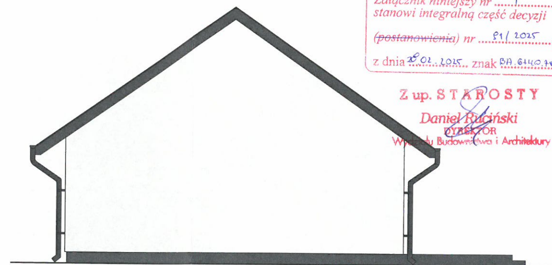
ELEWACJA PÓŁNOCNO-ZACHODNIA
