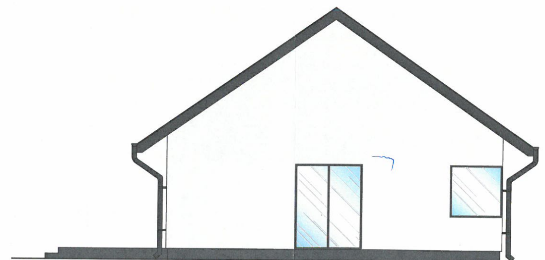
ELEWACJA POŁUDNIOWO-WSCHODNIA
