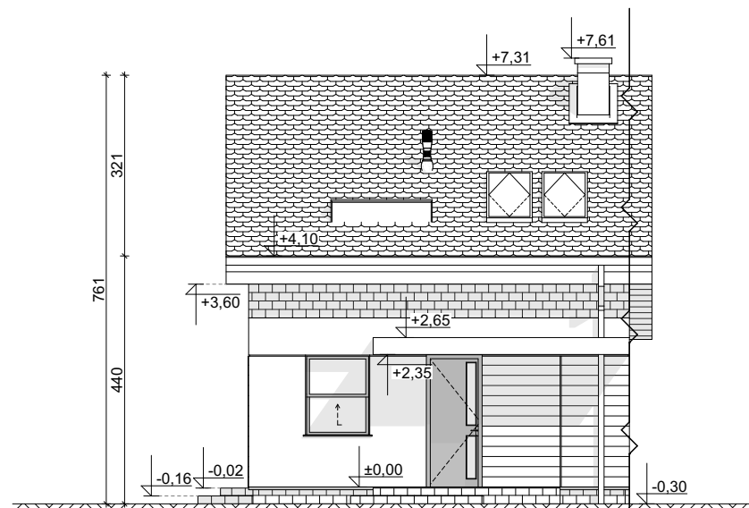
ELEWACJA FRONTOWA
