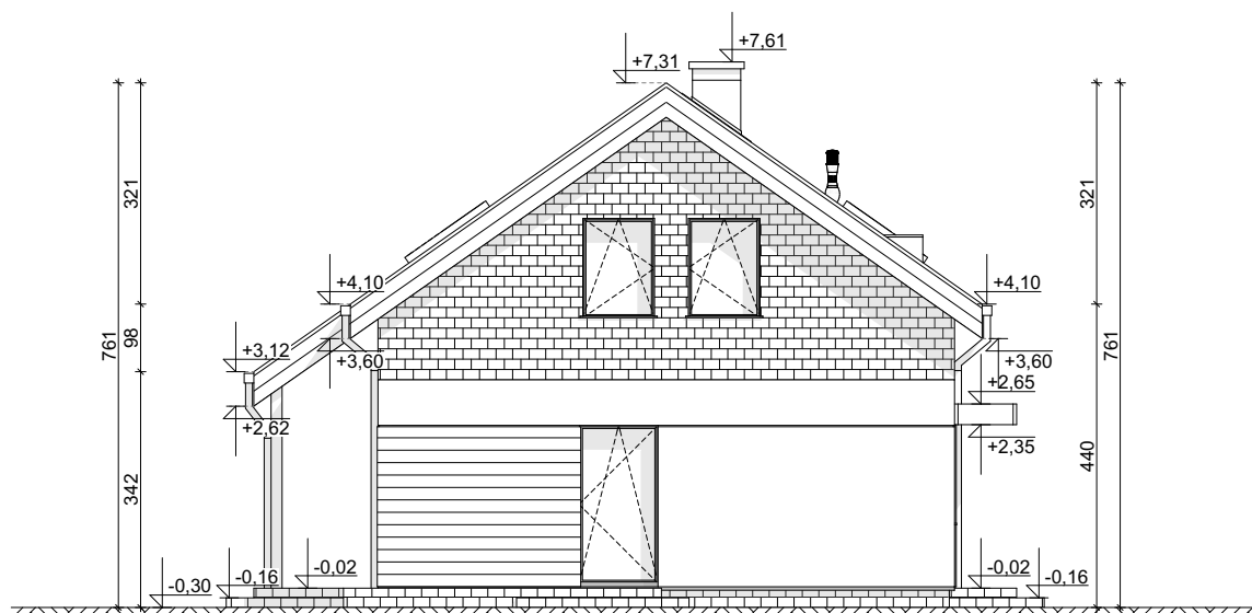
ELEWACJA BOCZNA
