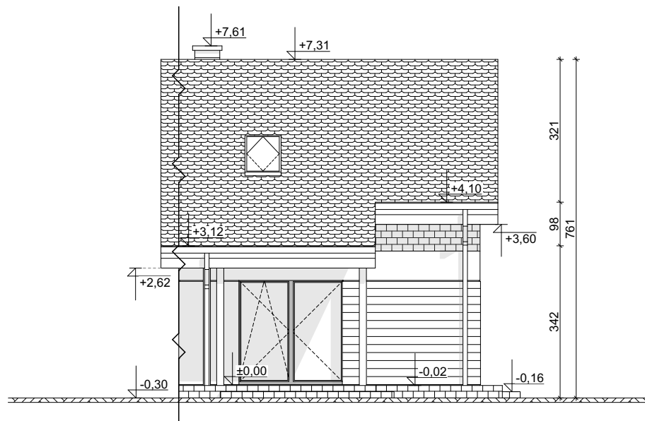
ELEWACJA OGRODOWA
